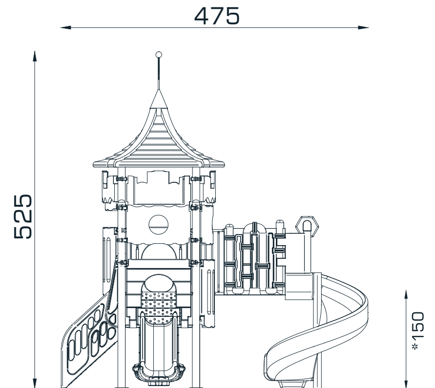
YAN GÖRÜNÜŞ / SIDE VIEW
