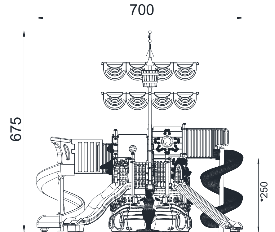
YAN GÖRÜNÜŞ / SIDE VIEW
