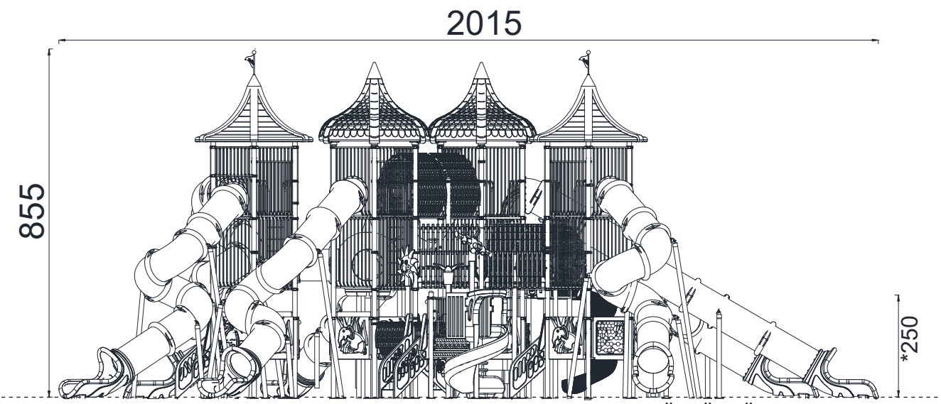
YAN GÖRÜNÜŞ / SIDE VIEW
