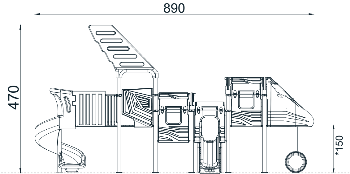
YAN GÖRÜNÜŞ / SIDE VIEW
