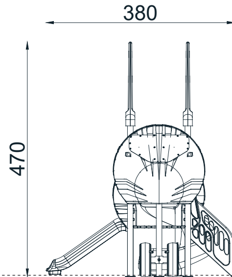
ÖN GÖRÜNÜŞ / FRONT VIEW
