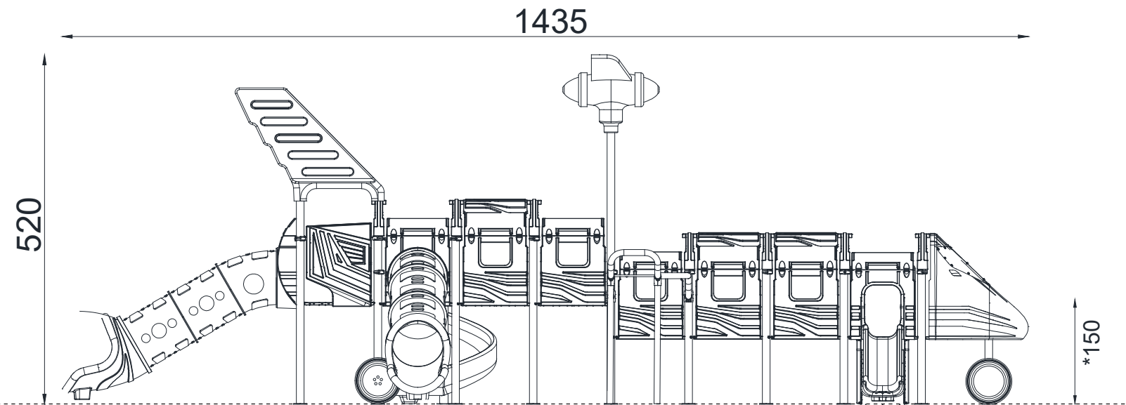
YAN GÖRÜNÜŞ / SIDE VIEW
