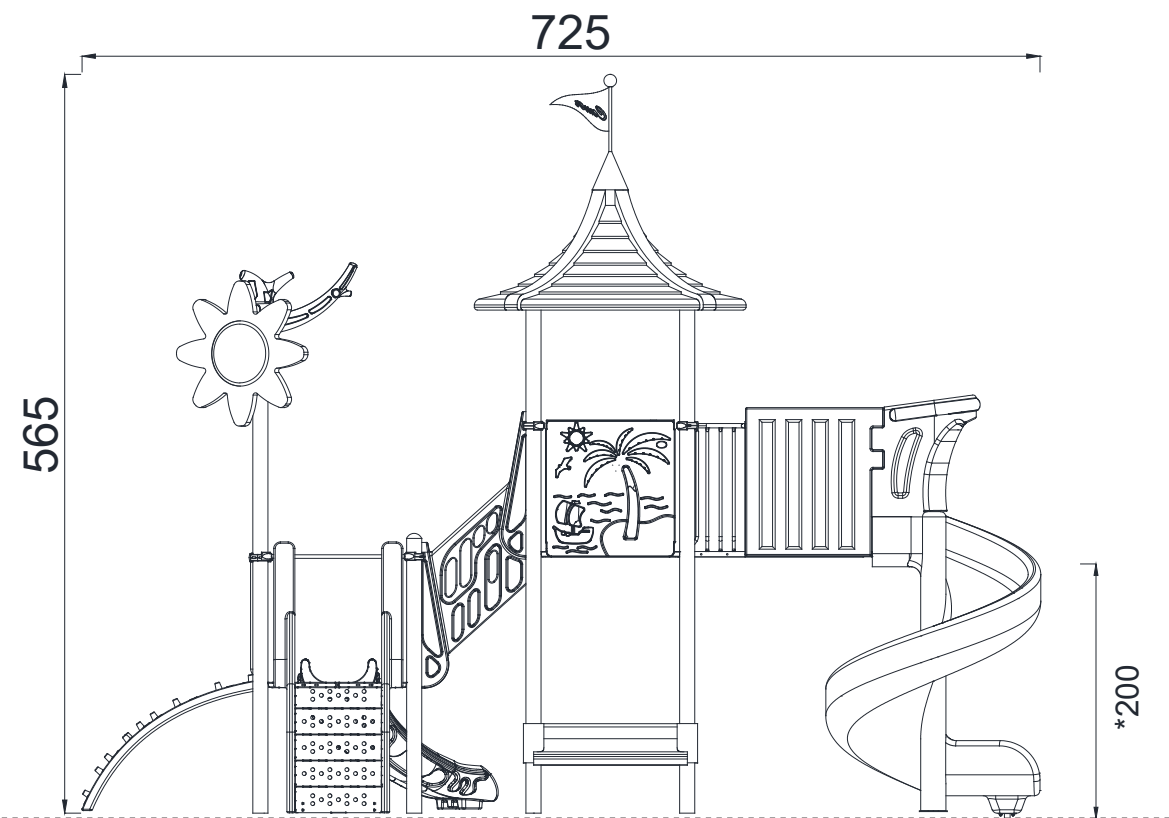
YAN GÖRÜNÜŞ / SIDE VIEW
