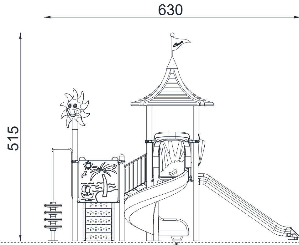
ÖN GÖRÜNÜŞ / FRONT VIEW
