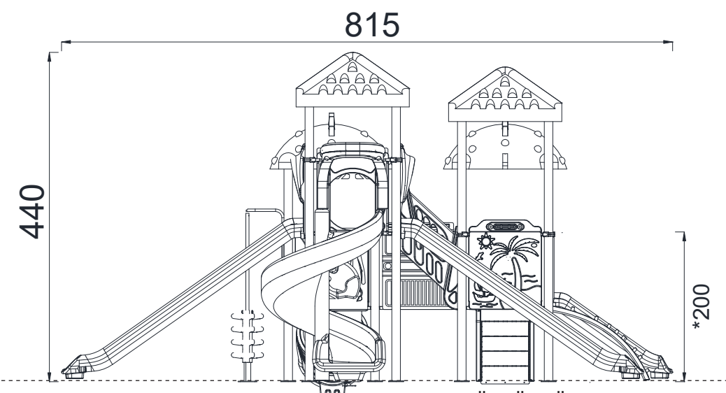
YAN GÖRÜNÜŞ / SIDE VIEW
