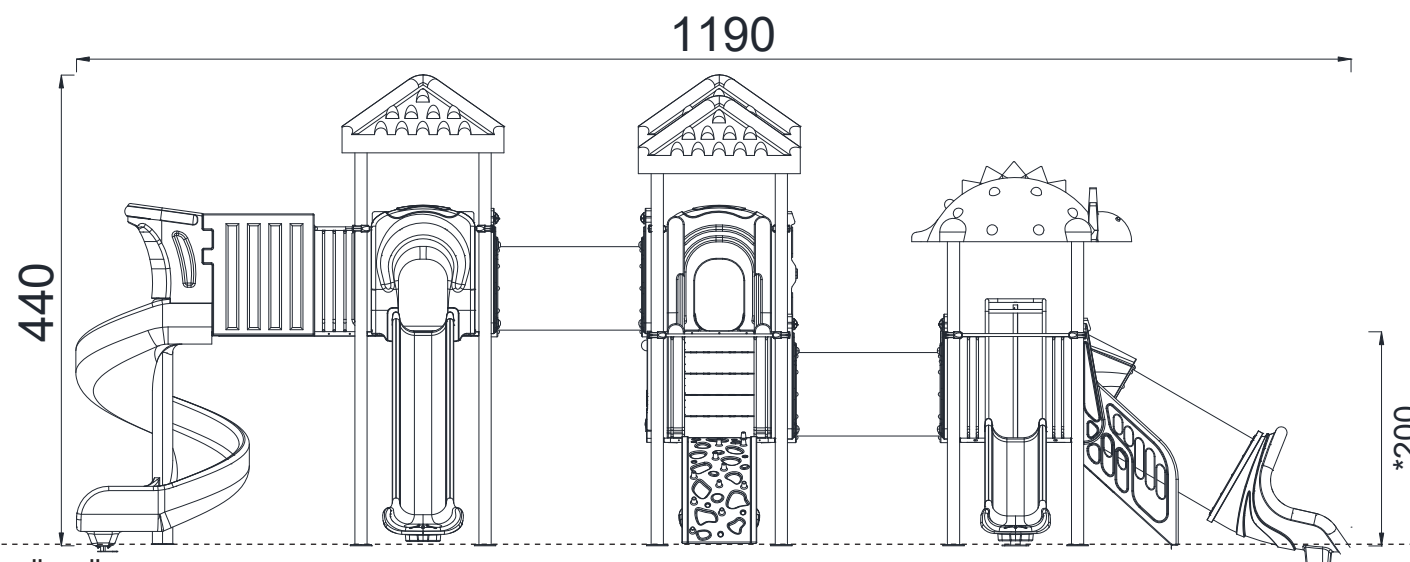
ÖN GÖRÜNÜŞ / FRONT VIEW
