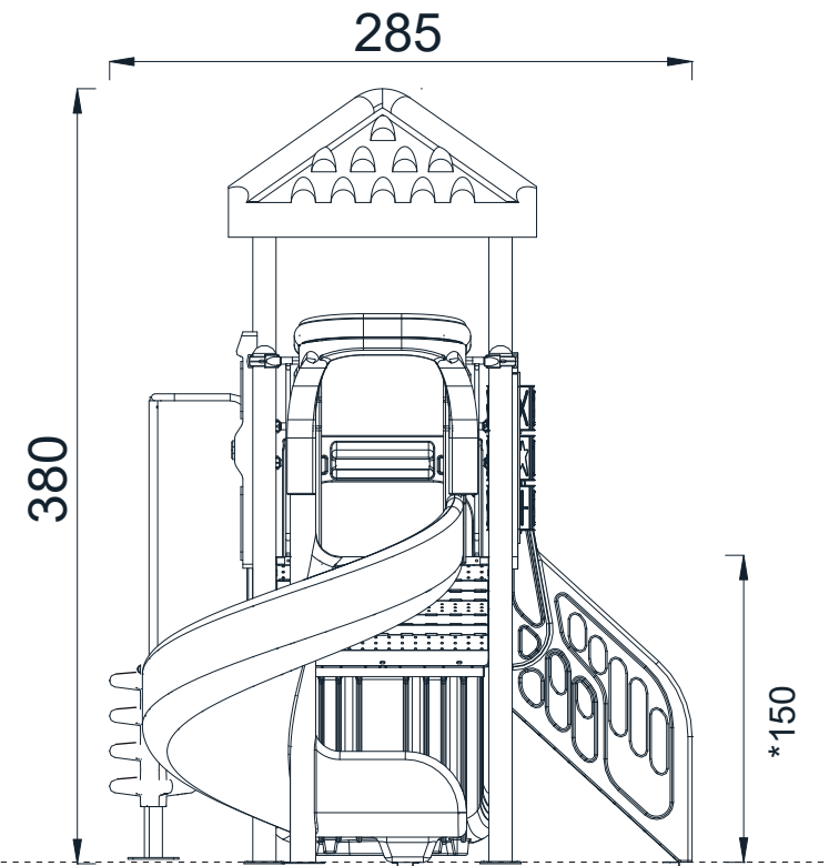
YAN GÖRÜNÜŞ / SIDE VIEW
