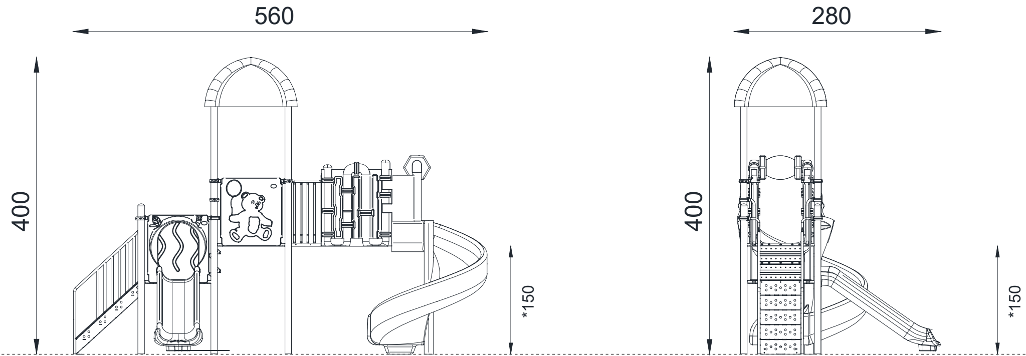
YAN GÖRÜNÜŞ / SIDE VIEW
