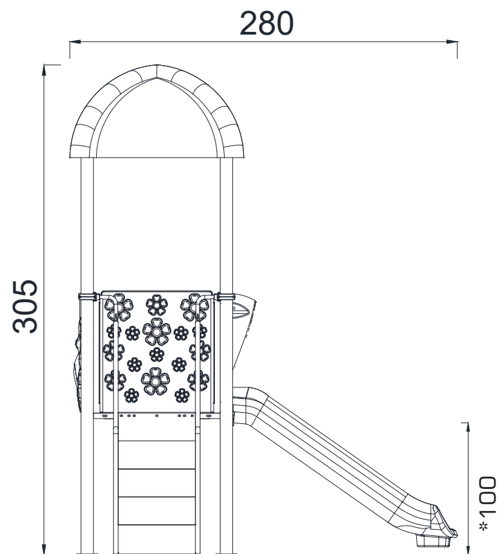
ÖN GÖRÜNÜŞ / FRONT VIEW
