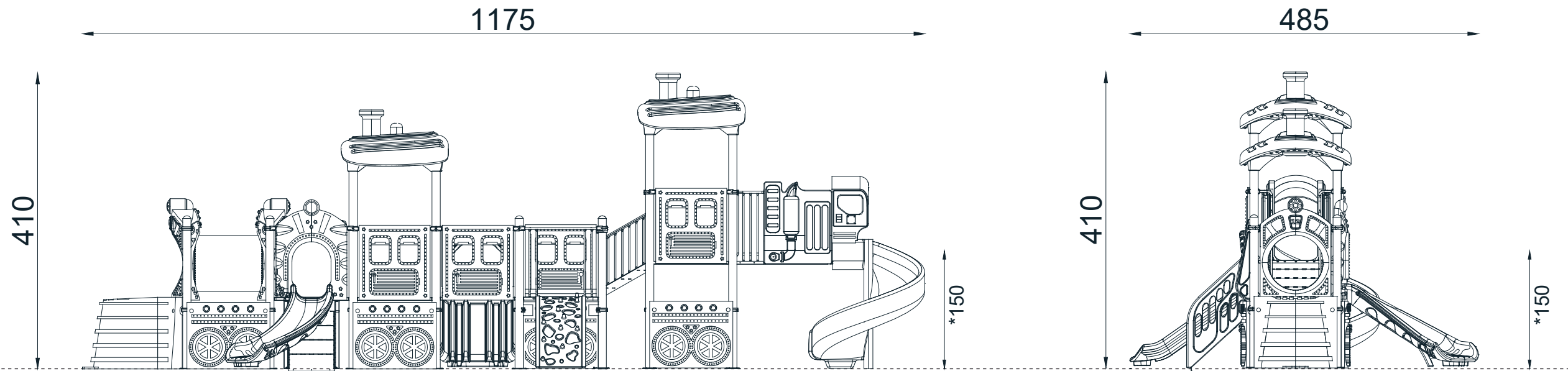
YAN GÖRÜNÜŞ / SIDE VIEW
